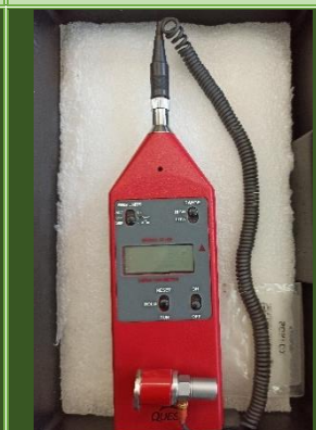
ارتعاش سنج سطوح مدل VT100
